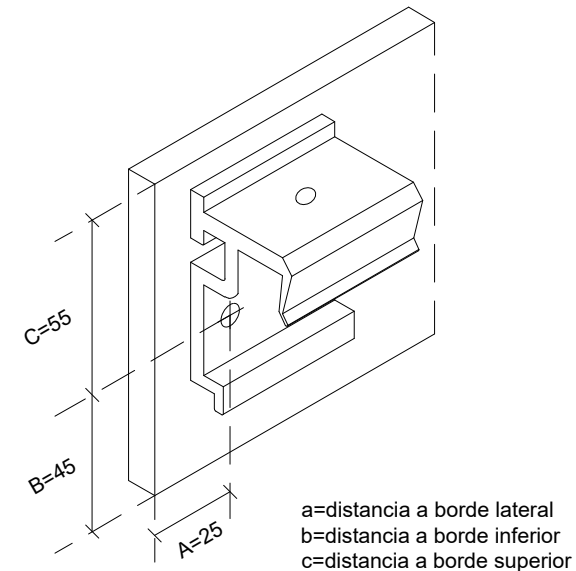
DETALLE FIJACIÓN COTAS EN MM
